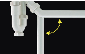
壁排水／床排水どちらにも対応可能な 直管トラップ。
