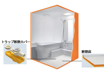
温熱環境対応断熱セット(カラリ床用)
